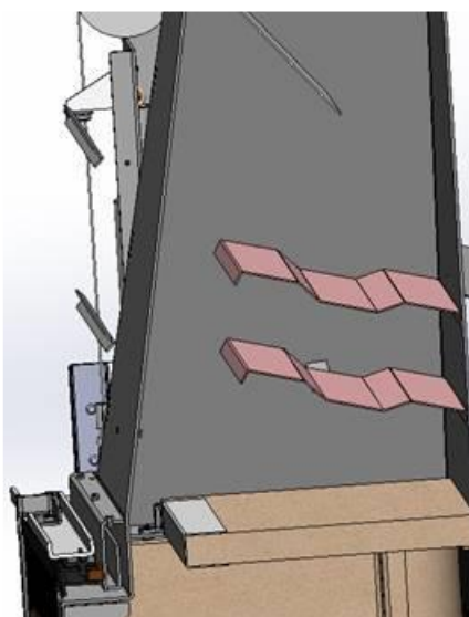
Figura n°28 - Cambio de posición del segundo deflector para evitar revoque.
