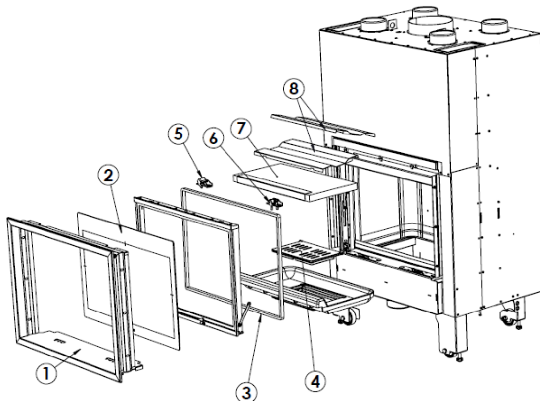
Figura nº42 - Despiece Itaca 80
