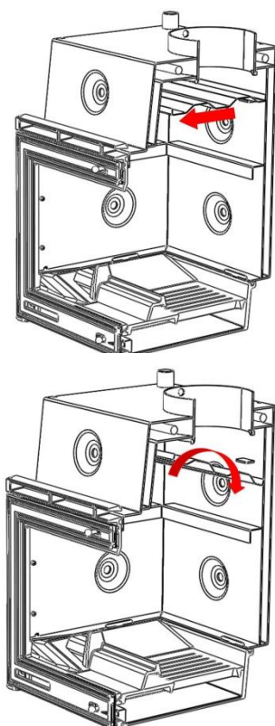
Figura nº18 - Desmontaje del deflector superior Sarria-Sakan 20
