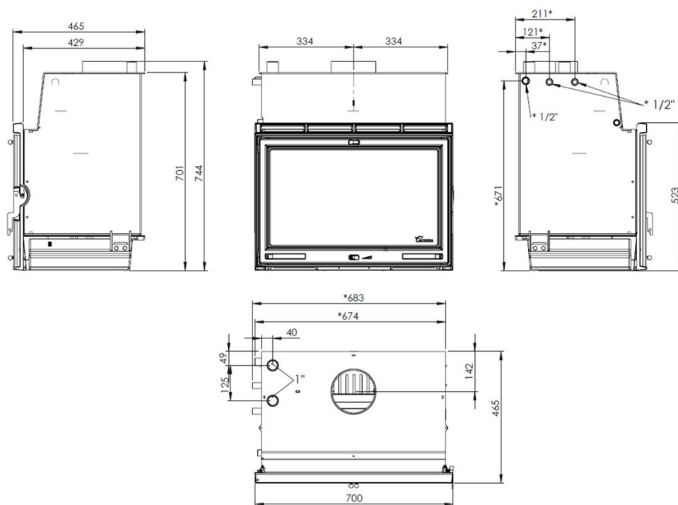
Figura nº1 - Dimensiones en mm del aparato SARRIA 6 - SAKAN 6
