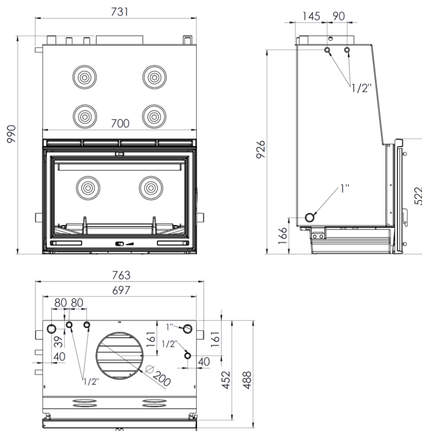
Figura nº5 - Dimensiones en mm del aparato SARRIA 16 - SAKAN 16
