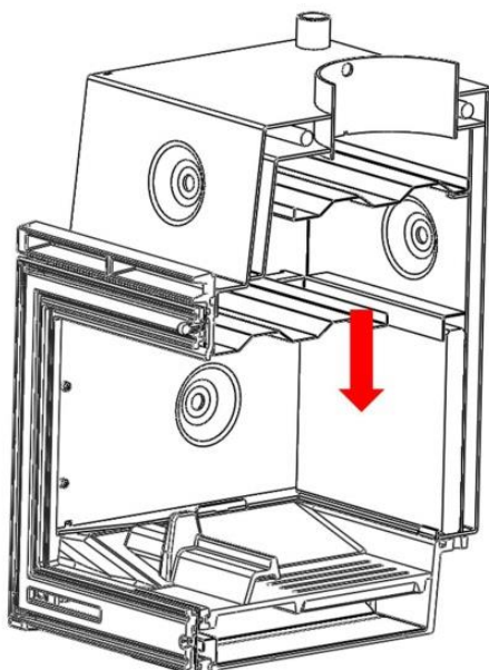
Figura n°9 - Meter la pieza girando y empujando hacia arriba hasta liberar la pestaña inferior y dejar caer
