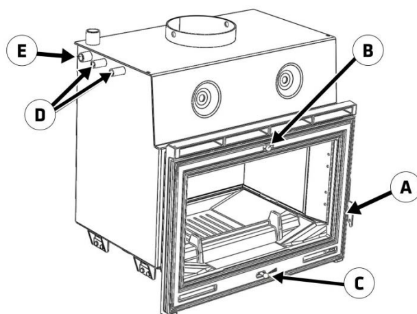
Figura n°17 - Elementos de funcionamiento del aparato
